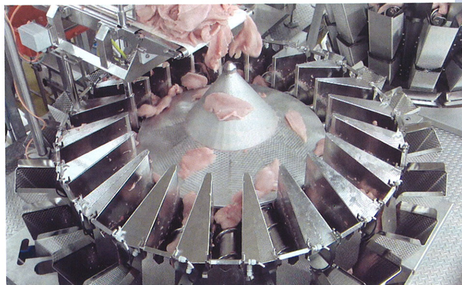
De såkaldte sensor gates på Cabinplant's multihead vejer minimerer "giv-væk" procenten i pakningerne
